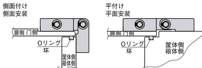
取付け例 FB-1736-A・B-3 安装例
