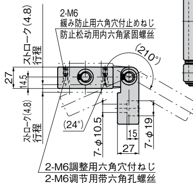
取付け例 FB-1736-A・B-3 安装例
