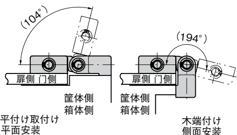
取付け例 FB-1736-A-1 安装例
