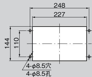
パネル穴明け寸法(1/2) 面板开孔尺寸(1/2)
