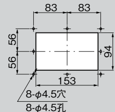
パネル穴明け寸法(1/2) 面板开孔尺寸(1/2)
