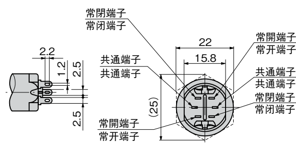
(2回路2接点型の裏面) (2电路2触点型的背面)
